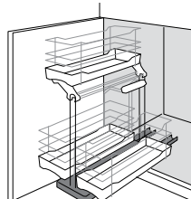
Kessebohmer Sink Caddy sku ex: SBCADDY3
